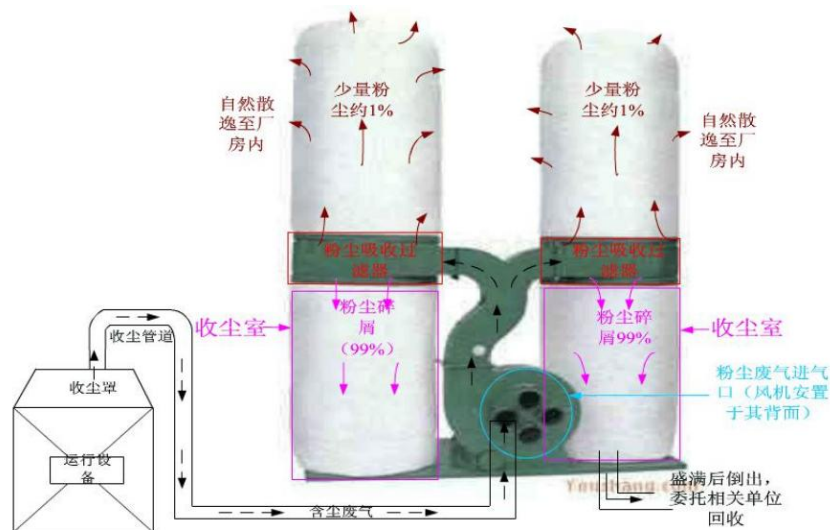
图 4-1 袋式除尘器工作示意图
