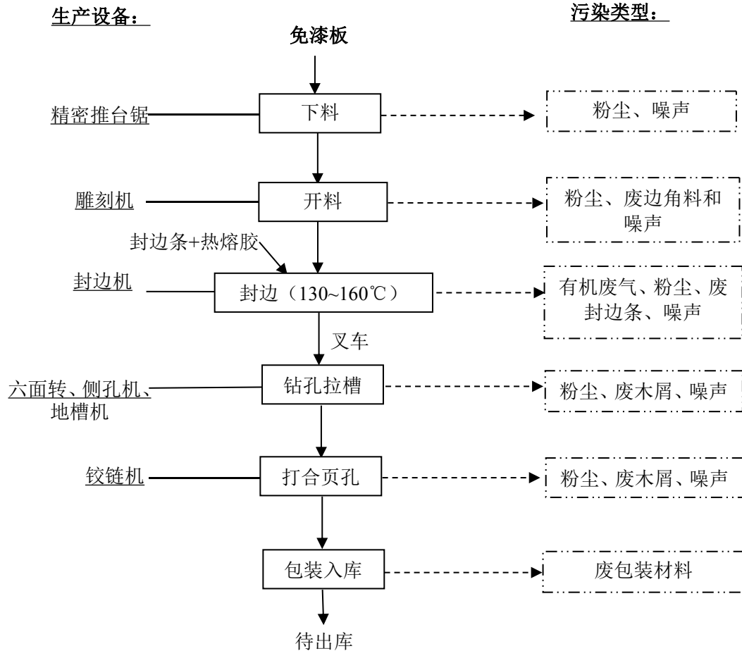
图 2-3 生产工艺流程及产污位置图
